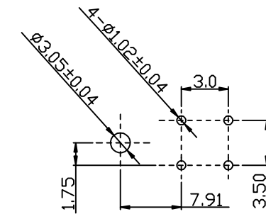
PCB板孔示意图
